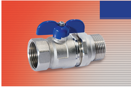
KOLLEKTÖR VANASI / VALVE FOR MANIFOLDS Вентиль коллектора с вентил коллектора / محبس مع شئوصل
